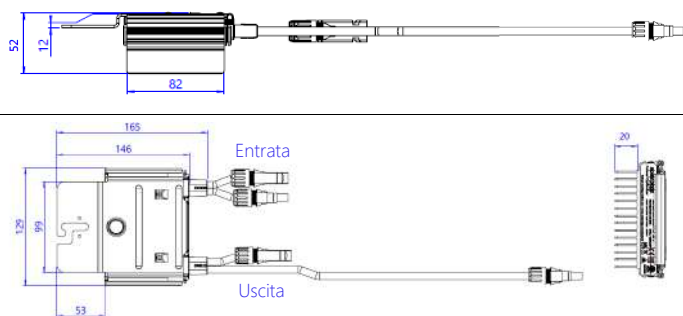
DISEGNO MECCANICO S1000
