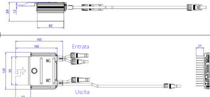
DISEGNO MECCANICO S1200
