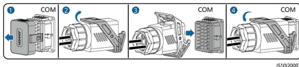
Figura 5-44 Fissaggio del connettore del cavo di segnale
