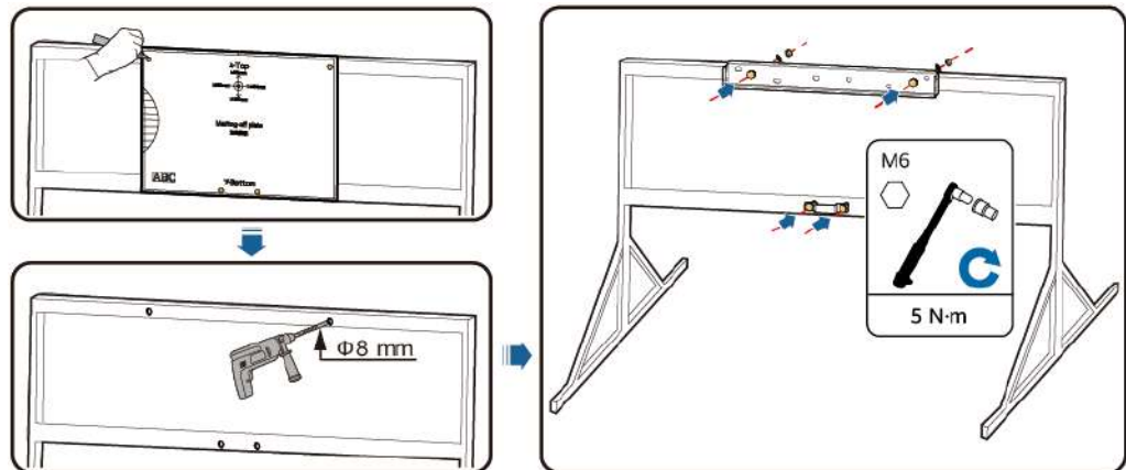
Figura 4-9 Fissaggio della staffa di montaggio
