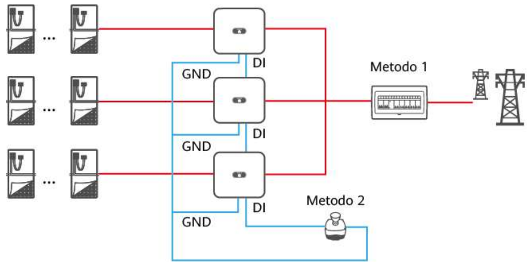
Figura C-1 Metodi di attivazione di un arresto rapido
