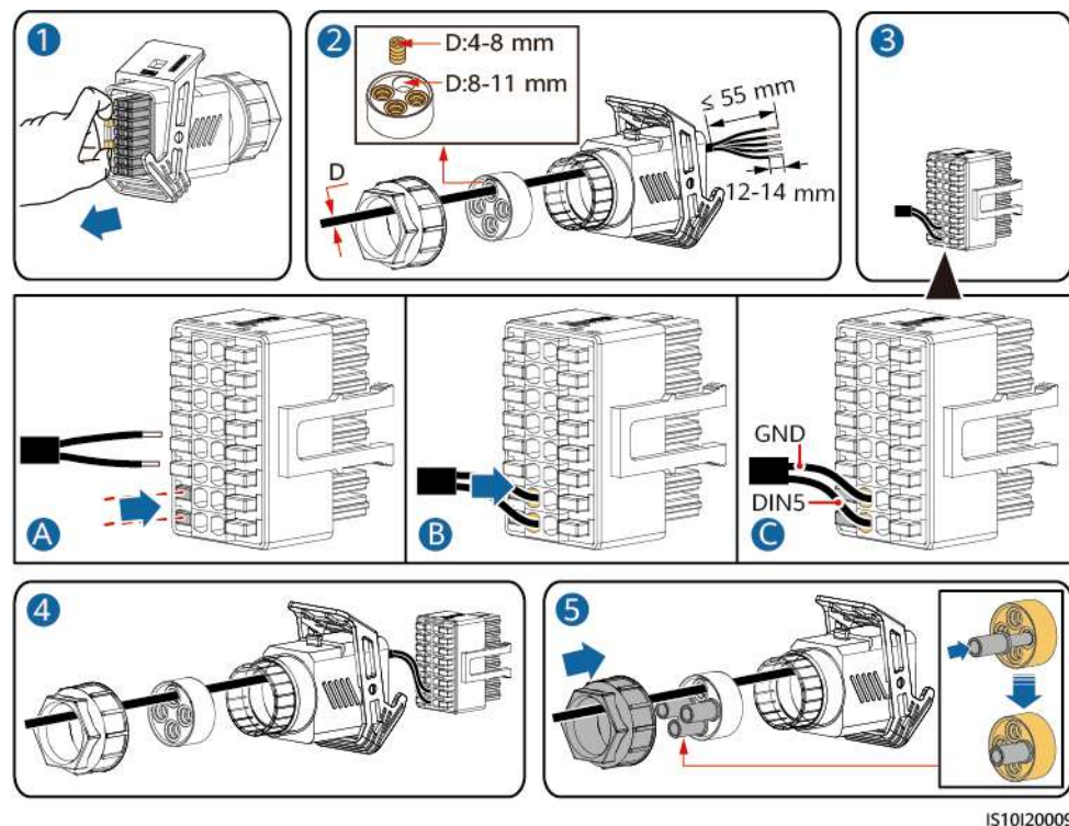
Figura 5-36 Installazione del cavo
