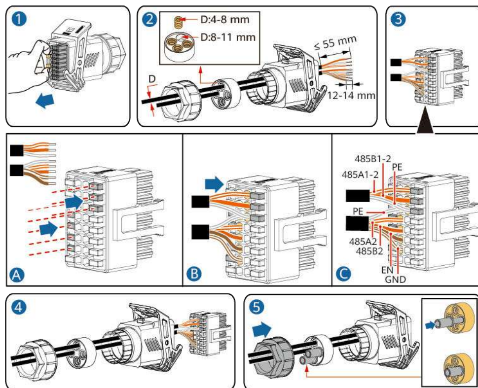
Figura 5-32 Installazione dei cavi
