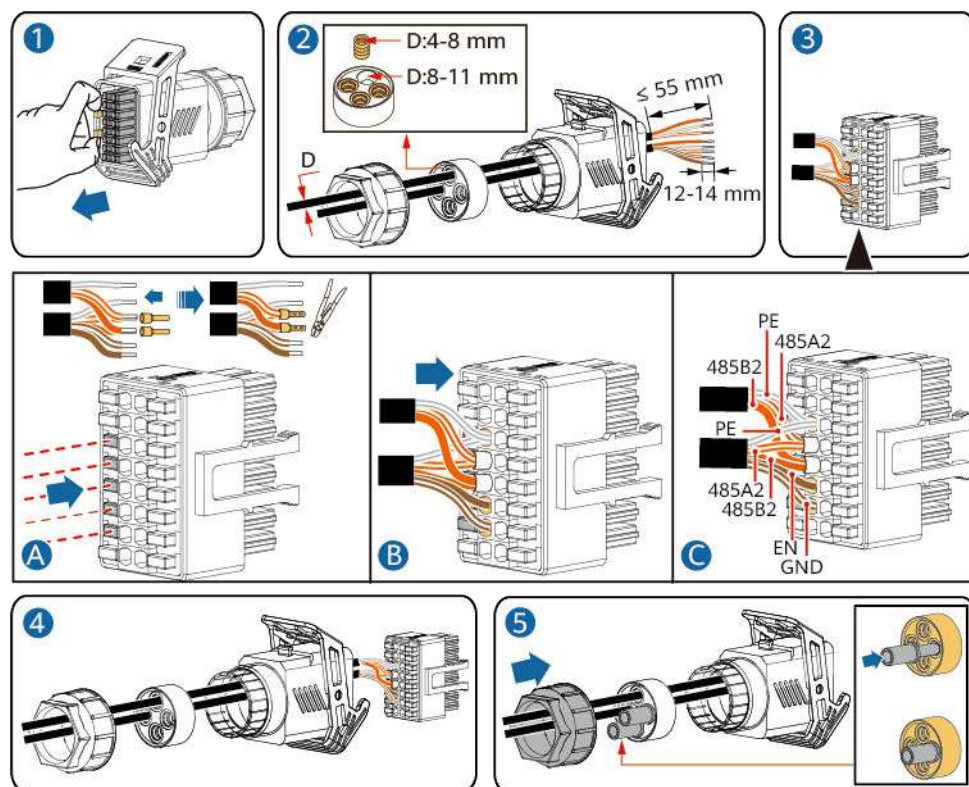
Figura 5-28 Installazione dei cavi
