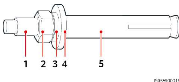
Figura 4-6 Struttura di un bullone a espansione M6
