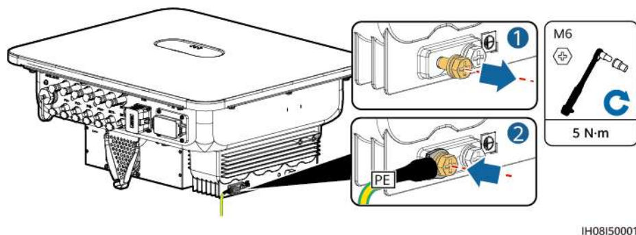
Figura 5-3 Collegamento del cavo PE
