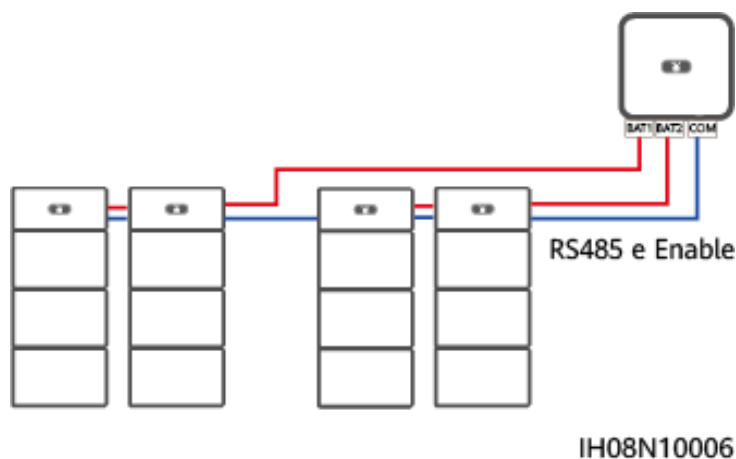
Figura 2-8 Collegamento dell'inverter a quattro batterie
