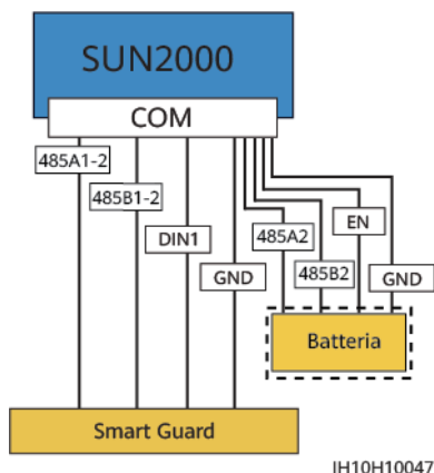
Figura 5-20 Connessione in rete di Smart Guard (i componenti nelle caselle tratteggiate sono opzionali)
