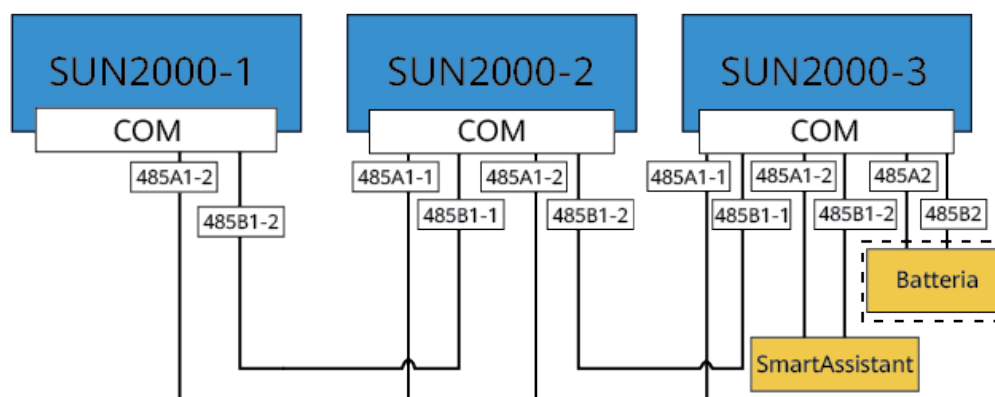
Figura 5-19 Connessione in rete di SmartAssistant (i componenti nelle caselle tratteggiate sono opzionali)
