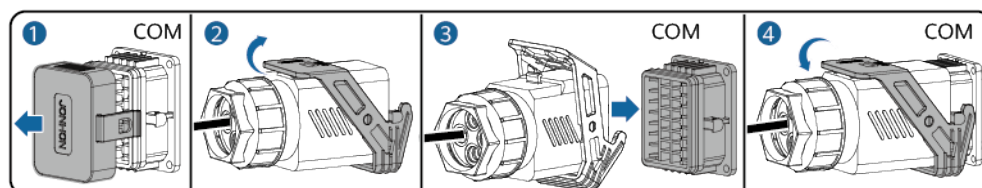
Figura 5-41 Fissaggio del connettore del cavo di segnale
