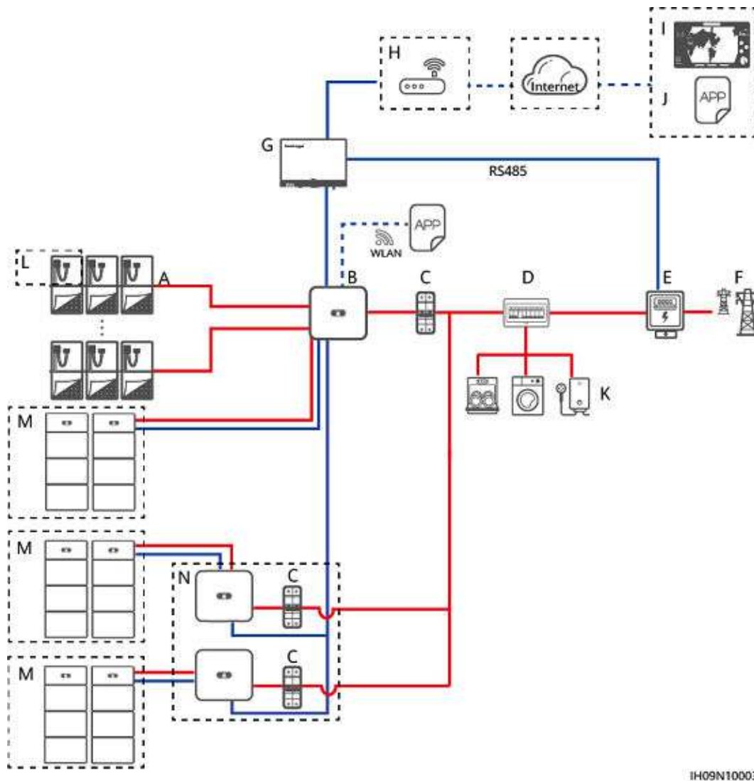
Figura 2-6 Collegamento in rete di SmartLogger (i componenti nelle caselle tratteggiate sono opzionali)
