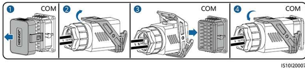
Figura 5-22 Fissaggio del connettore del cavo di segnale
