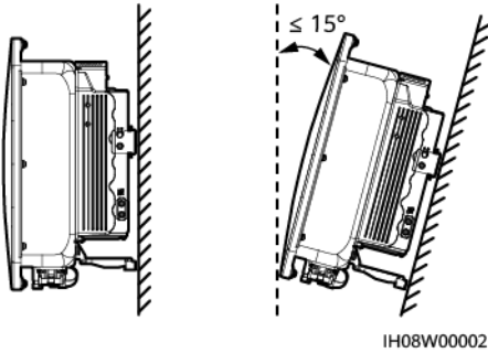
Figura 4-5 Angolo di installazione
