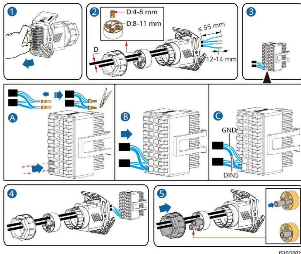
Figura 5-43 Installazione dei cavi
